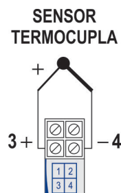
Fig. 9 – Conexiones eléctricas del transmisor (Termocupla)
