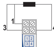
Fig. 7 – Conexiones eléctricas del transmisor (Pt100 3 hilos)
