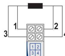
Fig. 8 – Conexiones eléctricas del transmisor (Pt100 4 hilos)
