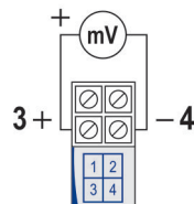
Fig. 10 – Conexiones eléctricas del transmisor (0-50 mV)
