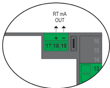
Figura 02 – Terminales de la retransmisión de PV (RT mA OUT)
